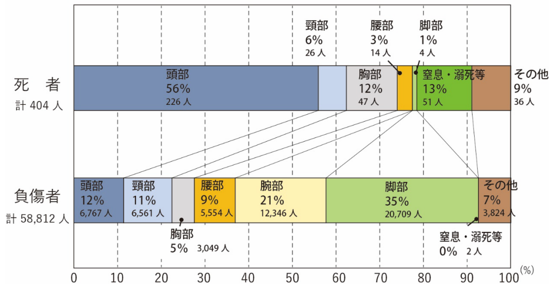
図 ヘルメット非着用の自転車乗車中死者・負傷者の人身損傷主部位別比較（令和2年）
